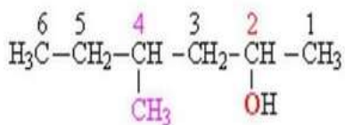
4-метилгексанол-2
