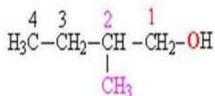
2-метилбутанол-1
